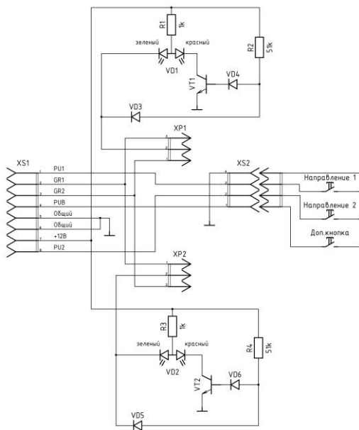
Схема электрическая принципиальная пульт дистанционный П2П-0-0Г
